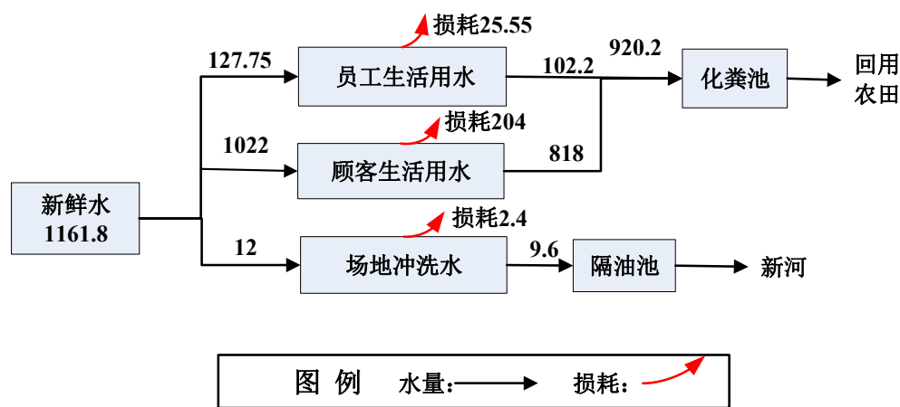
图 2-1 朝阳加油站水平衡图 (m³/a)
