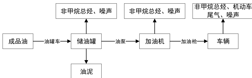
图 2-2 加油站工艺流程及产污环节图
