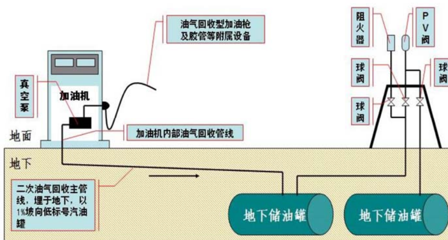
图 3-3 加油区油气回收（二次油气回收）系统基本原理图
