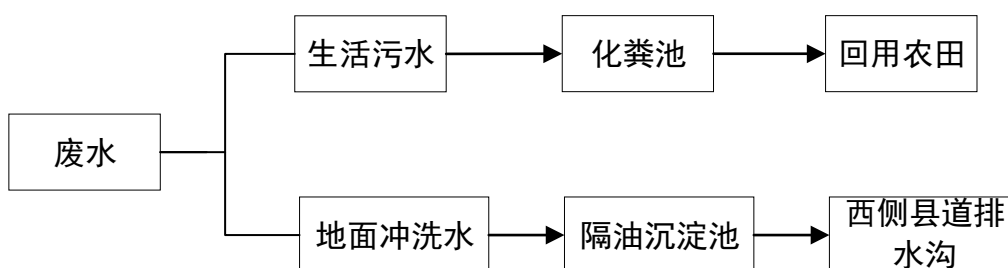
图 3-4 项目污水排放流程图
