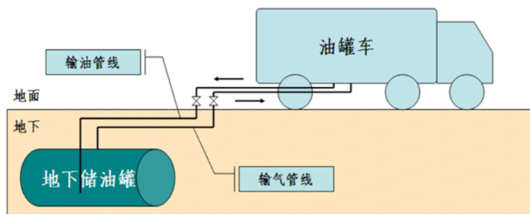
图 3-1 卸油区油气回收（一次油气回收）系统基本原理图
