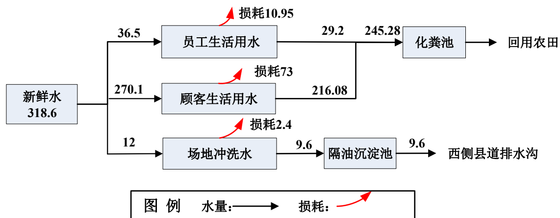
图 2-1 南坝加油站水平衡图 (m³/a)
