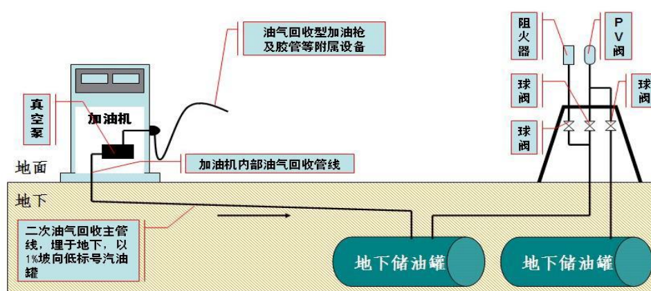
图 3-4 加油区油气回收（二次油气回收）系统基本原理图
