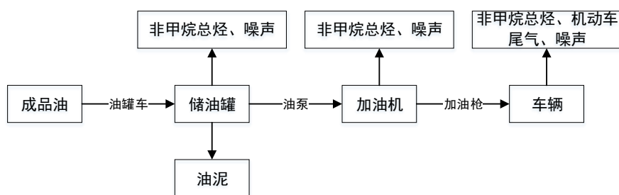
图 2-2 加油站工艺流程及产污环节图
