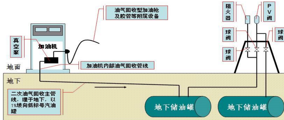
图 3-4 加油区油气回收（二次油气回收）系统基本原理图
