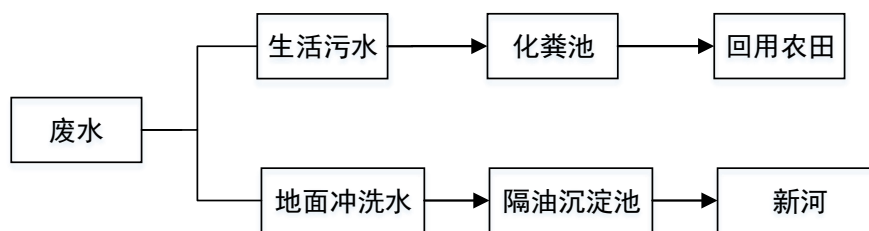
图 3-5 项目污水排放流程图
