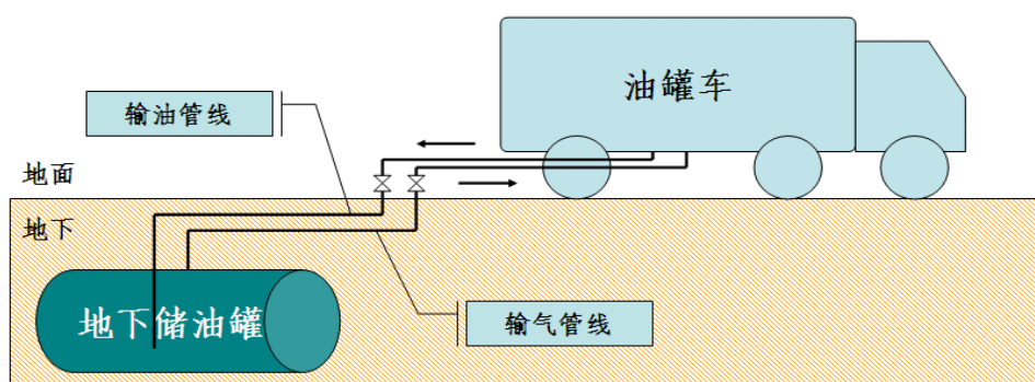
图 3-3 卸油区油气回收（一次油气回收）系统基本原理图
