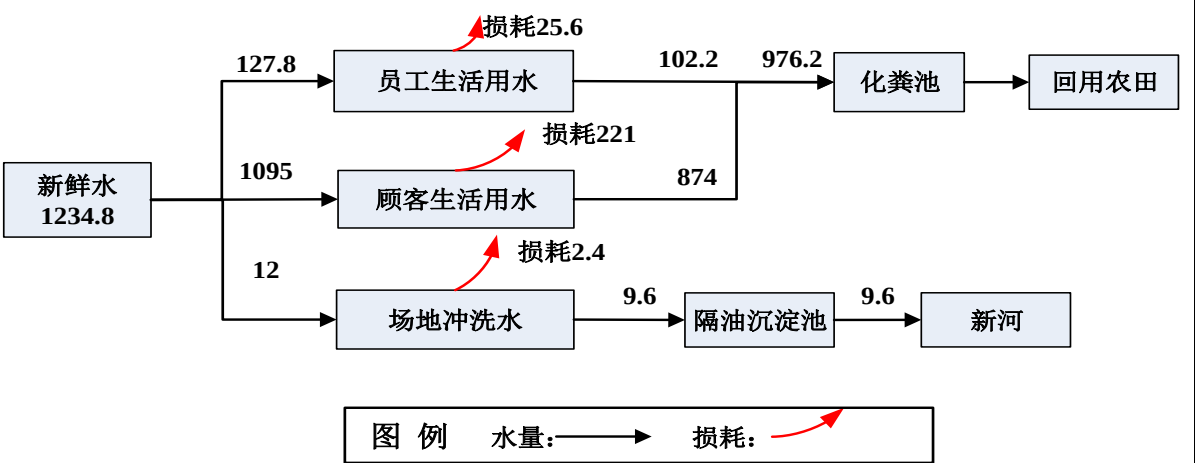
图 2-1 天龙加油站水平衡图 (m³/a)
