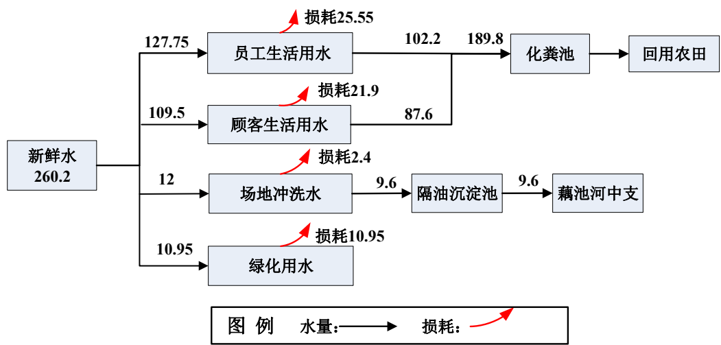
图 2-1 青华铺加油站水平衡图 (m³/a)
