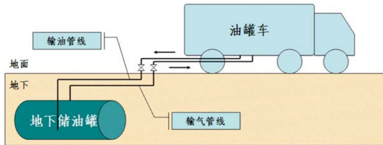
图 3-2 卸油区油气回收（一次油气回收）系统基本原理图
