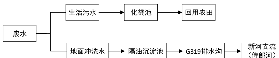
图 3-5 项目污水排放流程图
