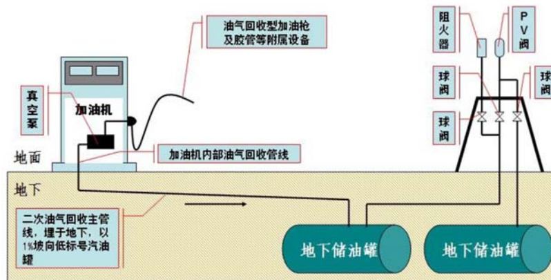
图 3-3 加油区油气回收（二次油气回收）系统基本原理图
