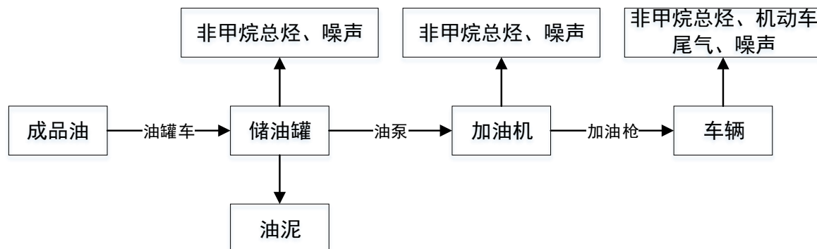
图 2-1 加油站工艺流程及产污环节图
