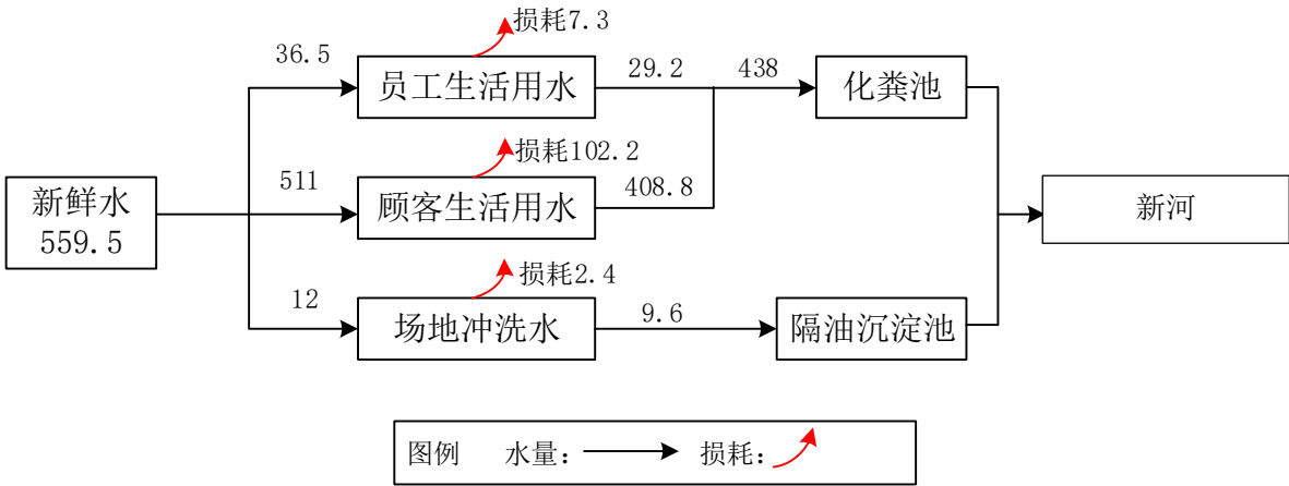
图 2-1 水平衡图 (m³/a)
