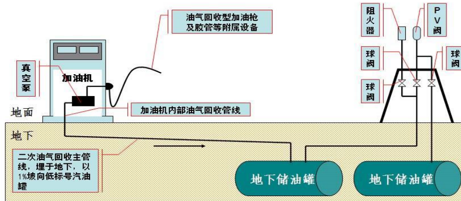
图 3-5 加油区油气回收（二次油气回收）系统基本原理图
