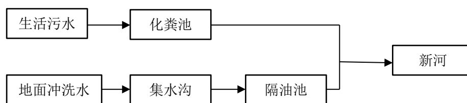
图 3-1 项目污水排放流程图
