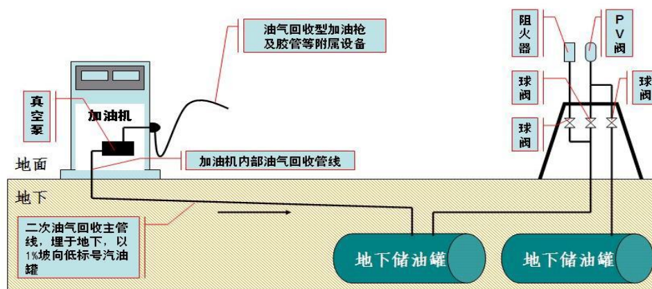
图 3-5 加油区油气回收（二次油气回收）系统基本原理图
