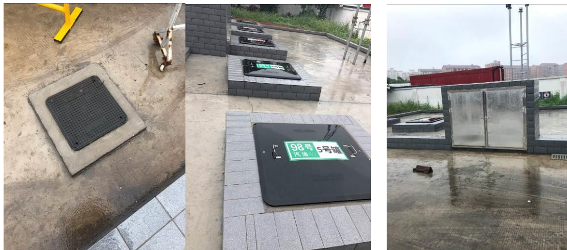
图 3-8 油罐区防渗、监测井
