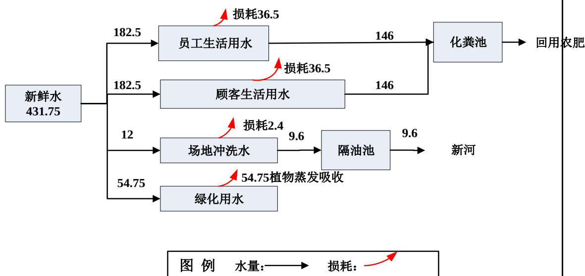
图 2-1 水平衡图 (m³/a)
