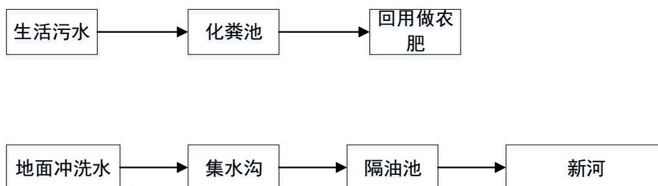
图 3-5 项目污水排放流程图
